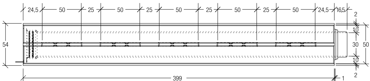
Draufsicht
